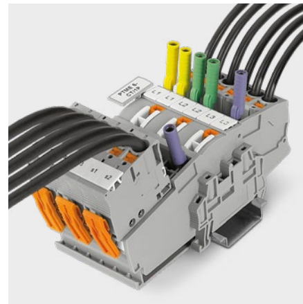
PTME 6/1P-Klemmen
