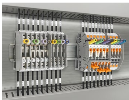
Mit den Messwandler-Trennklemmen bauen Sie Ihre Schaltanlagen platzsparend und modular auf. Die Messwandler-Trennklemmen sind in verschiedenen Anschlusstechniken erhältlich.
