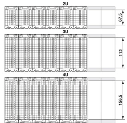
Höheneinheiten des FAME 3 RACK
