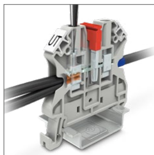
Reihen-klemme mit Schraubanschluss UT
