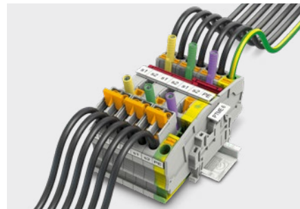
Messwandler-Trennklemmen PTME
