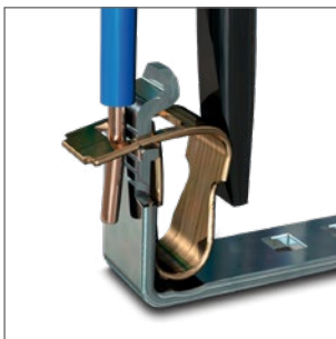
Klemmkörper einer Zugfederklemme
