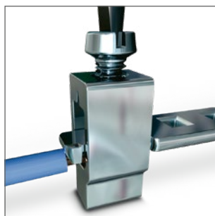
Anschlussprinzip einer Schraubklemme
