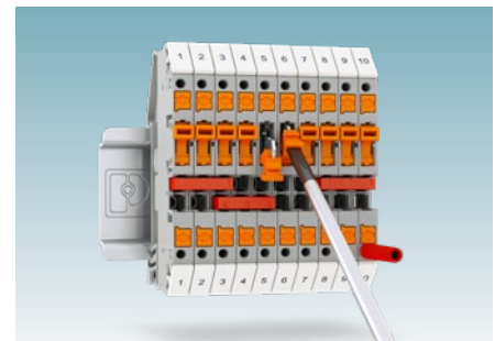
Messertrennklemmen PTV 2,5-MT
