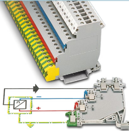
Sensor-/Aktor-Klemmen VIOK 1,5
