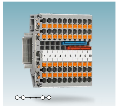
Mehrleiterklemmen PT 2,5-TWIN
