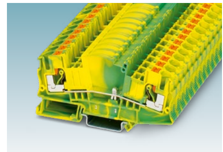
Schutzleiterklemme mit einem metallischen PE-Fuß
