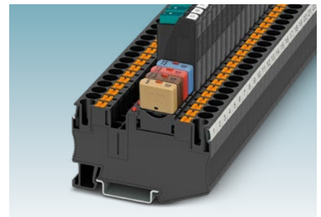
Thermische Schutzschalter für Überlast und Kurzschlusschutz
