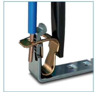
Klemmkörper einer Zugfederklemme
