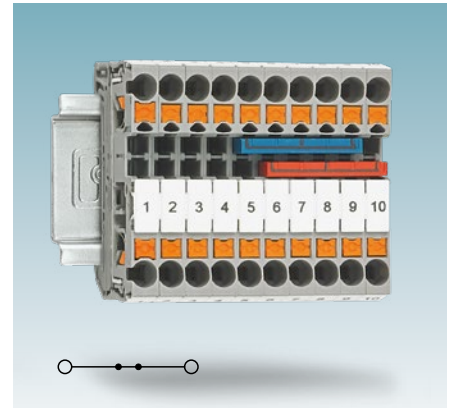
Durchgangsklemmen PT 2,5
