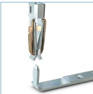
Klemmkörper einer steckbaren Klemme
