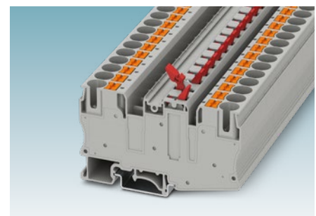
Hebel-Messertrennklemmen PT 10-MTL
