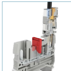
Reihenklemme ST 2,5/2P
