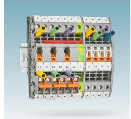
Wandlerklemmen UT
