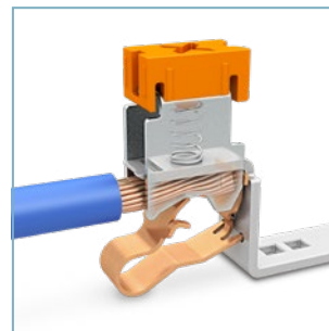
Klemmkörper einer XTV-Klemme
