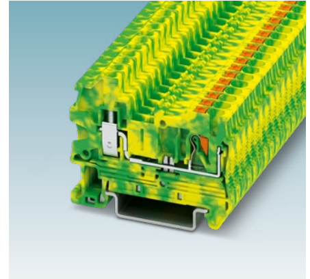
Schutzleiterklemme mit einem metallischen PE-Fuß
