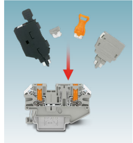
Trennklemme mit Trenn-, Sicherungs- und Bauelementestecker sowie Durchgangsverbinder
