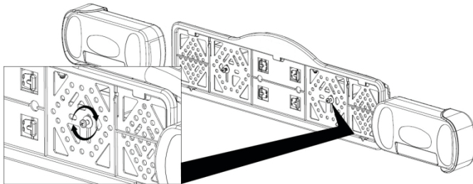
Bild 5: Montage Kennzeichenhalter
