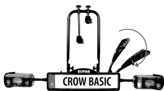
3. Dépliage des rails de roues de droite
