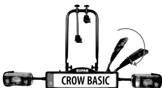
3. Ausklappen der rechten Radschienen
