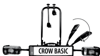
3. Apertura dei binari di destra
