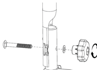
Figure 3 : Fixation de l'étrier en U
