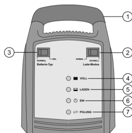
Illustration 1 : Vue avant
