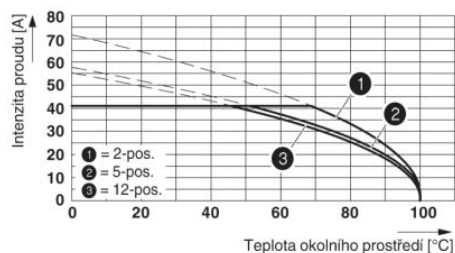
Zátěžová křivka pro: IPC 5/...-ST-7,62 s PC 5/...-ST-7,62 Průřez vodiče = 10 mm 2
