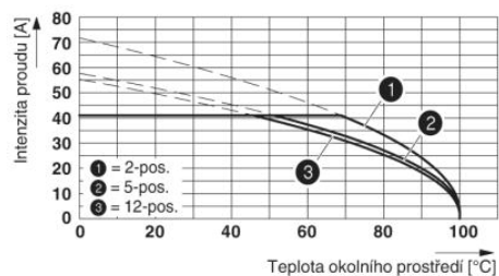
Zátěžová křivka pro: IPC 5/...-ST-7,62 s IPC 5/...-G-7,62 Průřez vodiče = 10 mm 2
