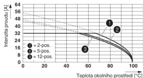
Zátěžová křivka pro: PC 5/...-ST1-7,62 s PC 5/...-G-7,62 Průřez vodiče: 6 mm 2
