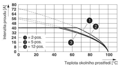
Zátěžová křivka pro: PC 5/...-ST1-7,62 s PC 5/...-G-7,62 Průřez vodiče: 10 mm 2
