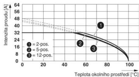
Zátěžová křivka pro: PC 5/...-ST1-7,62 s PCV 5/...-G-7,62 Průřez vodiče: 6 mm 2
