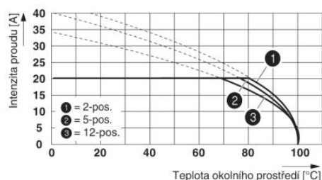
Zátěžová křivka pro: PC 5/...-ST1-7,62 s PCV 4/...-G-7,62 Průřez vodiče: 4 mm 2
