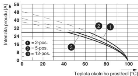
Zátěžová křivka pro: PC 5/...-ST1-7,62 s PC 4/...-G-7,62 Průřez vodiče: 4 mm 2
