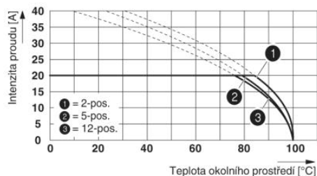
Zátěžová křivka pro: PC 5/...-ST1-7,62 s PCV 4/...-G-7,62 Průřez vodiče: 6 mm 2
