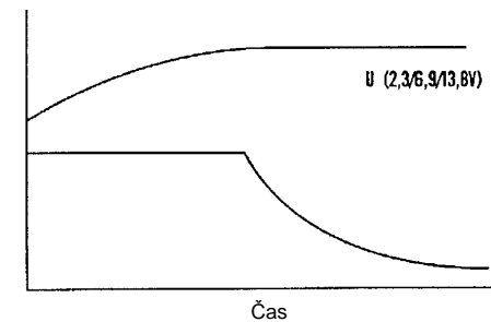
Nabíjecí charakteristika AL 300
