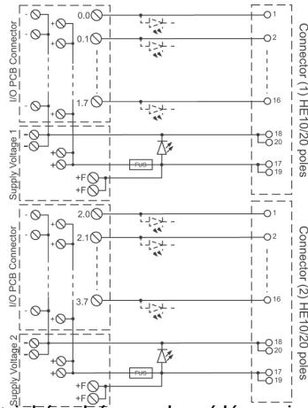
Elektrické schéma odpovídá verzi s LED.
