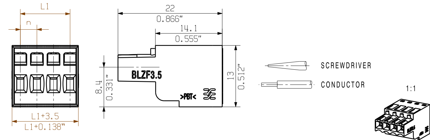
SHOWN:BLZF 3.50/04/180
