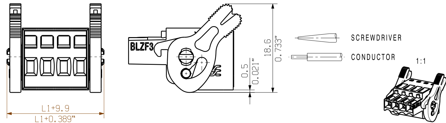
SHOWN:BLZF 3.50/04/180LR
