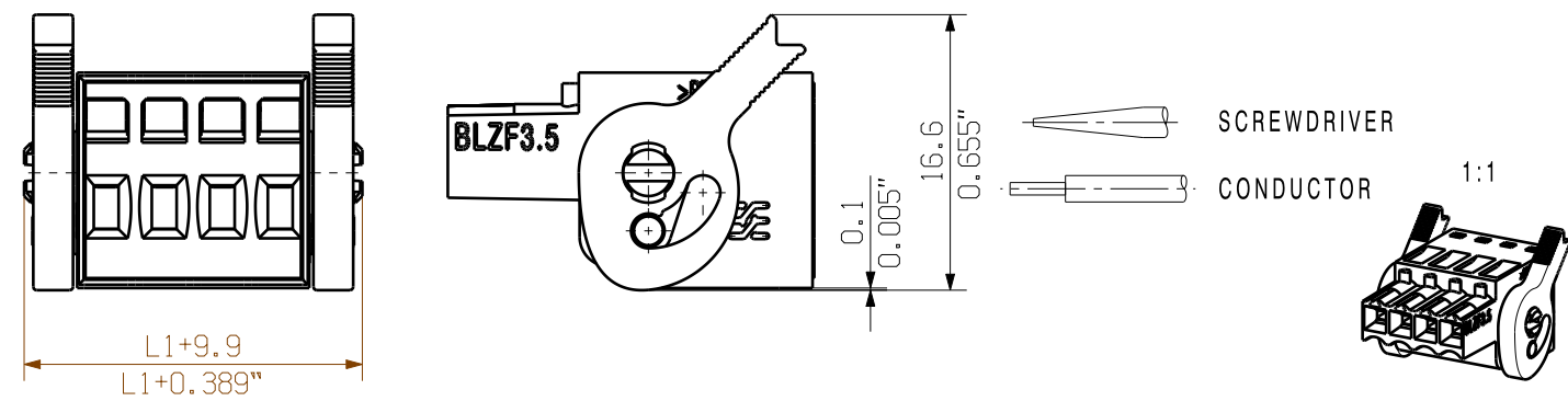
SHOWN:BLZF 3.50/04/180LH
