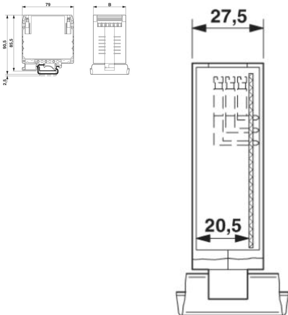
UEGM 25... a UEGM 27,5-SMD s 1 deskou plošných spojů, 6 pólů, resp. 12 pólů (FS/FS)
