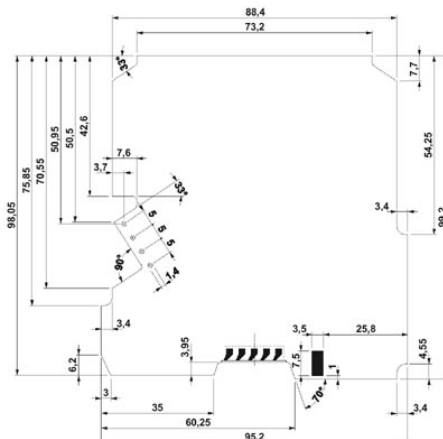
Schéma s rozměry desky plošných spojů ME MAX U-U1 pro techniku připojení svorek pro plošné spoje (MKDSO), pohled: strana osazení
