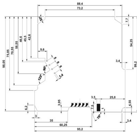
Schéma s rozměry desky plošných spojů ME MAX U-U1 pro techniku zástrčky (MSTBO), pohled: strana osazení
