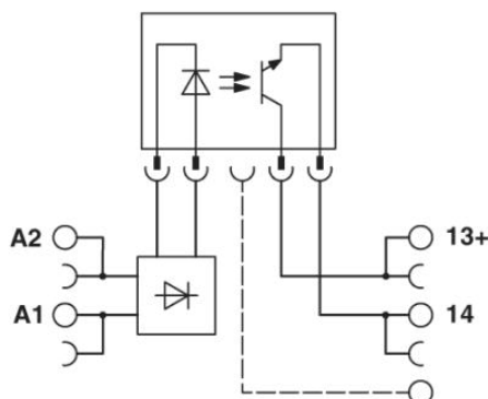
Schéma zapojení
