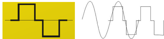
Modifikovaný sinusový průběh výstupního střídavého napětí 230 V
