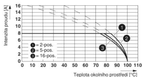
Typ: MC 1,5/...-STF-3,81 s DFK-MC 1,5/...-GF-3,81 (s pájeným spojem)
