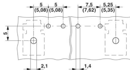
Vodorovně ležící zásuvka konektoru
