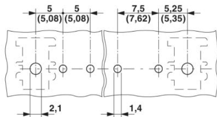
Svisle stojící zásuvka konektoru
