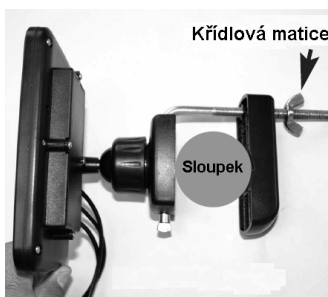
Montáž na sloupek (stožár)
