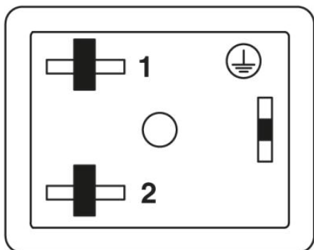
Obsazení pólů konektoru ventilu, konstrukce BI
