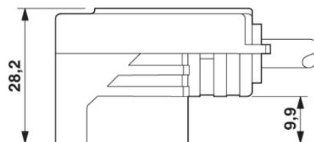
Konektor ventilu, provedení BI, pohled ze strany
