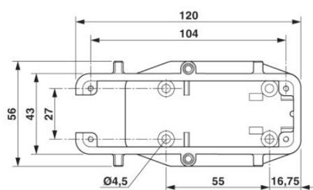
Rozměrový výkres, pohled shora
