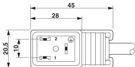
konektor ventilu, konstrukce B
