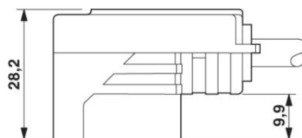
Konektor ventilu, provedení B, pohled ze strany
