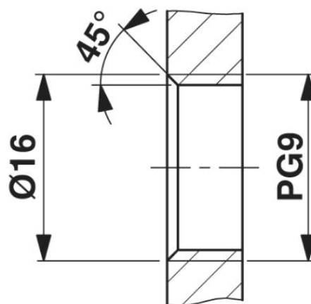
Výřez v pouzdru pro upevňovací závit Pg9, montážní stěna se závitem
