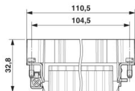
Kolíková vložka
