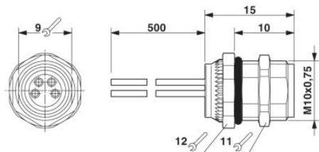
Vestavná zásuvka M8
