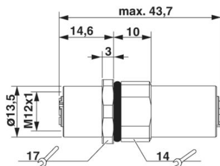
Průchodka rozvaděče, oboustranná přípojka M12
