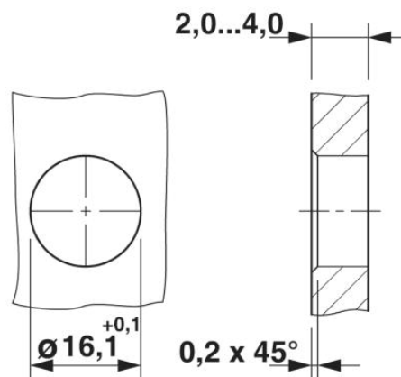
Montážní otvor
