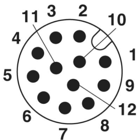
Obsazení pólů zástrčky M12, 12pólová, pohled ze strany kolíku
