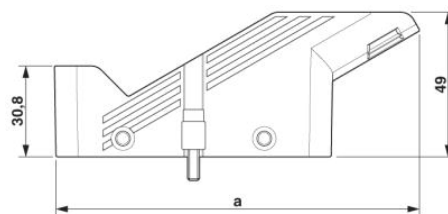
Rozměrový výkres, a=150,2mm
