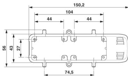
Rozměrový výkres, pohled shora
