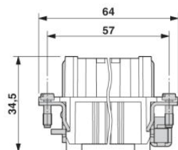
Zdírková vložka
