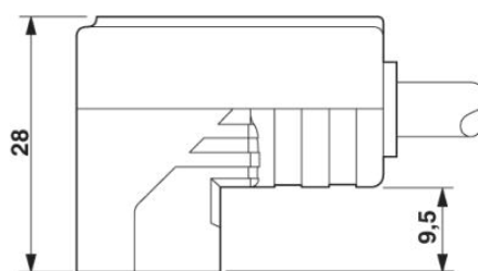
Konektor ventilu, provedení C, pohled z boku
