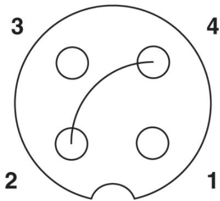
Obsazení pólů zdířky M12, 3pólové, PIN 2+4 přemostěný, s kódováním A, pohled ze strany zdířky
