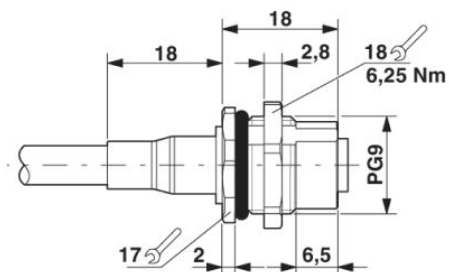
Stěnová průchodka M12
