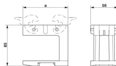
Rozměrový výkres, a=93,5mm
