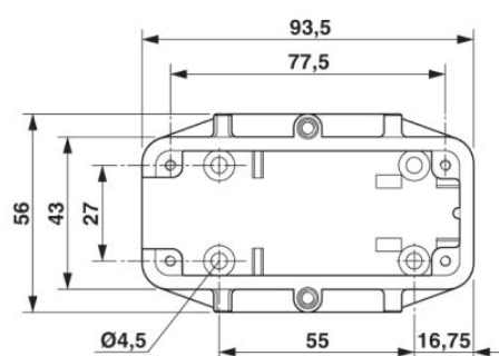
Rozměrový výkres, pohled shora
