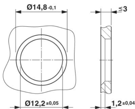
Výřez v pouzdru pro dvoudílné vestavné spojky (nebo vestavná spojka) M12, s THR a vlnovým pájeným spojem, varianta 1
