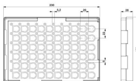
Balení THR-Tray
