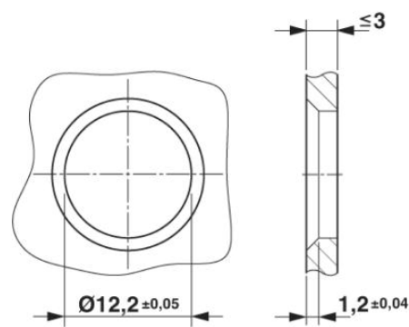
Výřez v pouzdru pro dvoudílné vestavné spojky (nebo vestavná spojka) M12, s THR a vlnovým pájeným spojem, varianta 2
