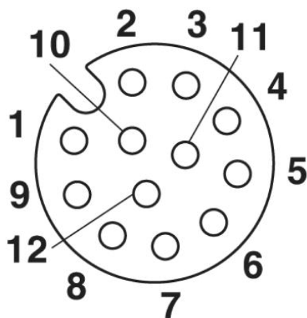
Obsazení pólů zástrčky M12, 12pólová, pohled ze strany zástrčky
