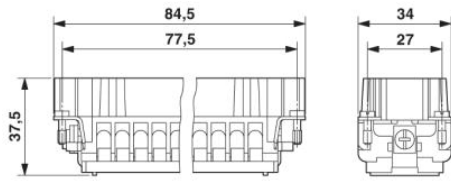
Kolíková vložka
