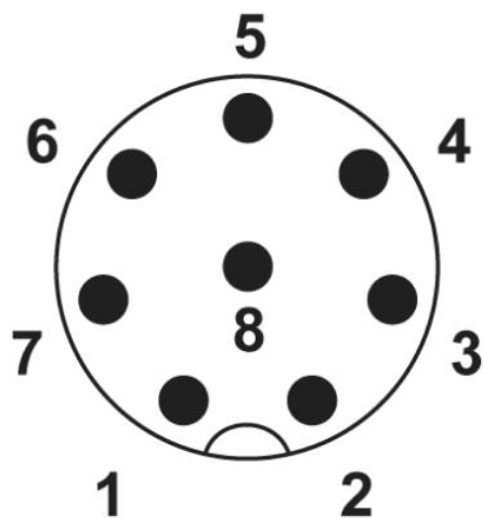
Obsazení pólů zástrčky M12, 8pólová, s kódováním A, pohled ze strany kolíku
