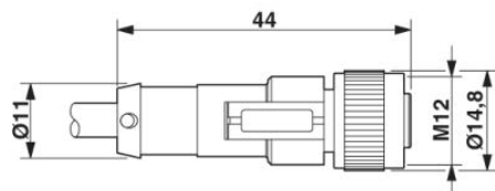
Zástrčka M12 x 1, rozbočovač Y
