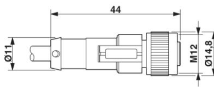
přímá zásuvka M12 x 1
