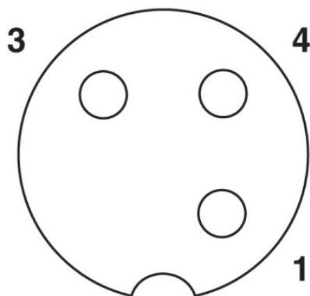
Obsazení pólů zdíčky M12, 3pólové, s kódováním A, pohled ze strany zdíčky
