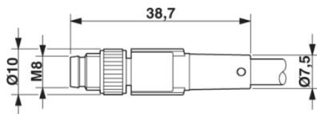
Zástrčka M8 x 1, přímá, stíněná
