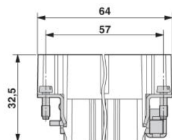
Kolíková vložka
