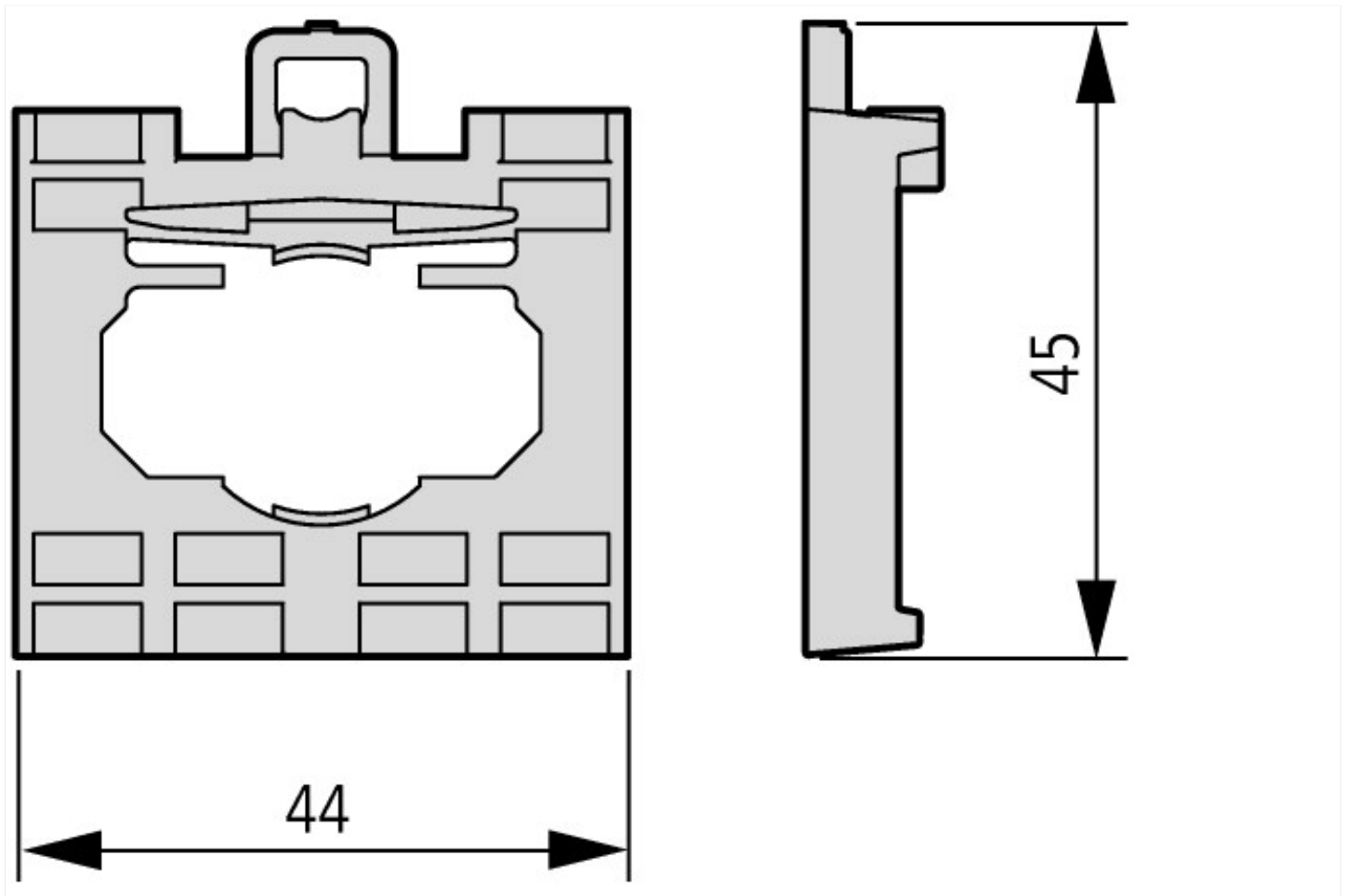
Upevňovací adaptér upevňovací adaptér (čelní montáž) pro 4
