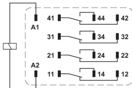
Schéma zapojení
