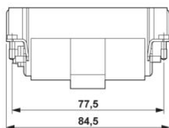
Rozměrový výkres
