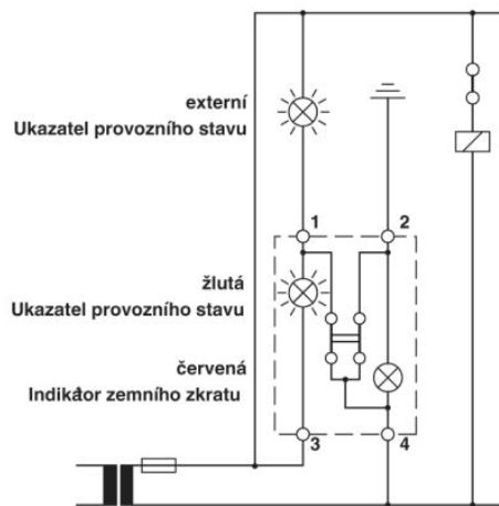
Uzemněný provozní stav
