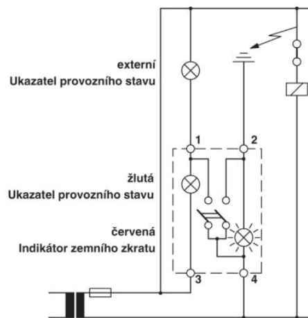
Případ zemního zkratu
