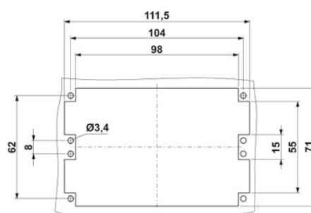
Montážní otvor
