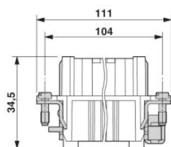
Zdírková vložka
