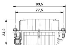
Zdířková vložka
