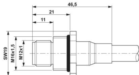
Vestavná zástrčka M12
