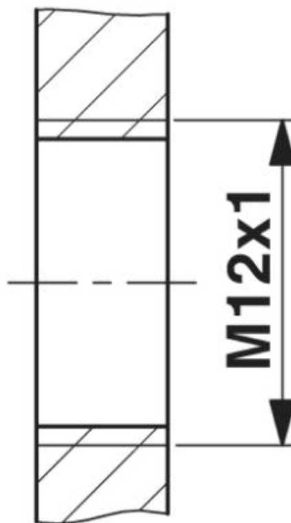
Výřez v pouzdru pro upevňovací závit M12, montážní stěna se závitem
