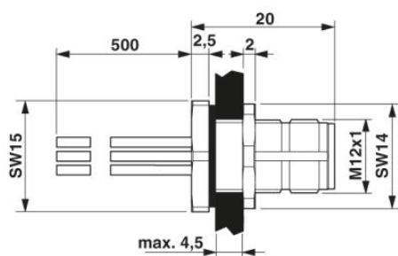
M12 přídatný zástrčkový spoj
