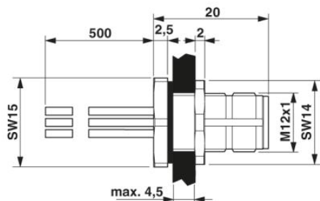
M12 přídavný zástrčkový spoj
