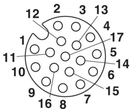
Obsazení pólů zástrčky M12, 17pólová, pohled ze strany zástrčky
