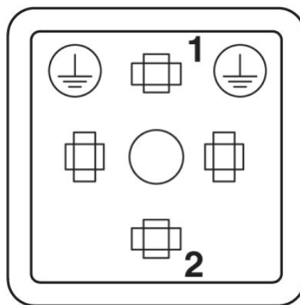
Obsazení pólů konektoru ventilu, konstrukce CI
