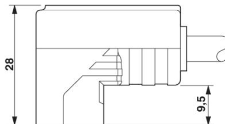
Konektor ventilu, provedení CI, pohled ze strany
