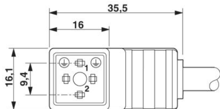
konektor ventilu, konstrukce CI
