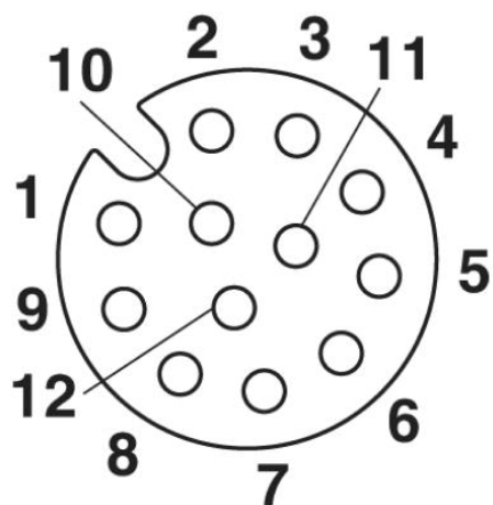
Obsazení pólů zástrčky M12, 12pólová, pohled ze strany zástrčky
